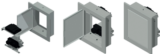
Rys. 6. Montaż sterownika gazu wraz z odbiornikiem w skrzynce rozdzielczej
